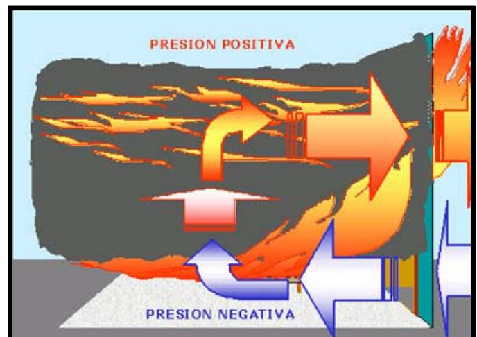
Imagen 5: Esquema del flujo de ventilación en un flashover.
